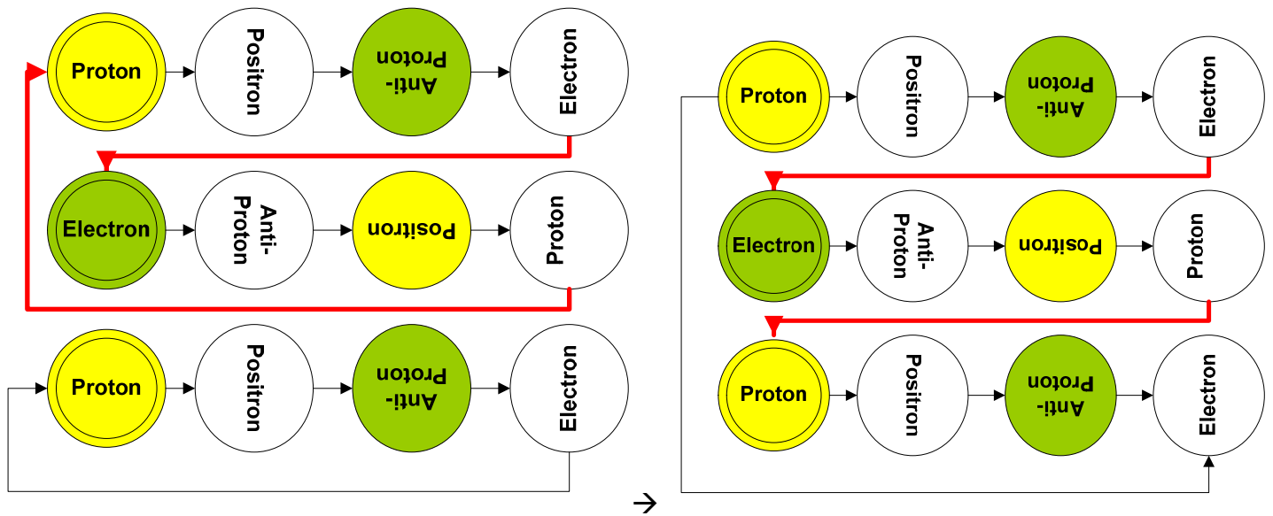
Figure 32. Deuterium diagram.
