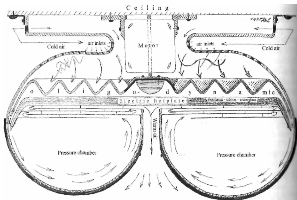
Fig. 28: The Klimator
